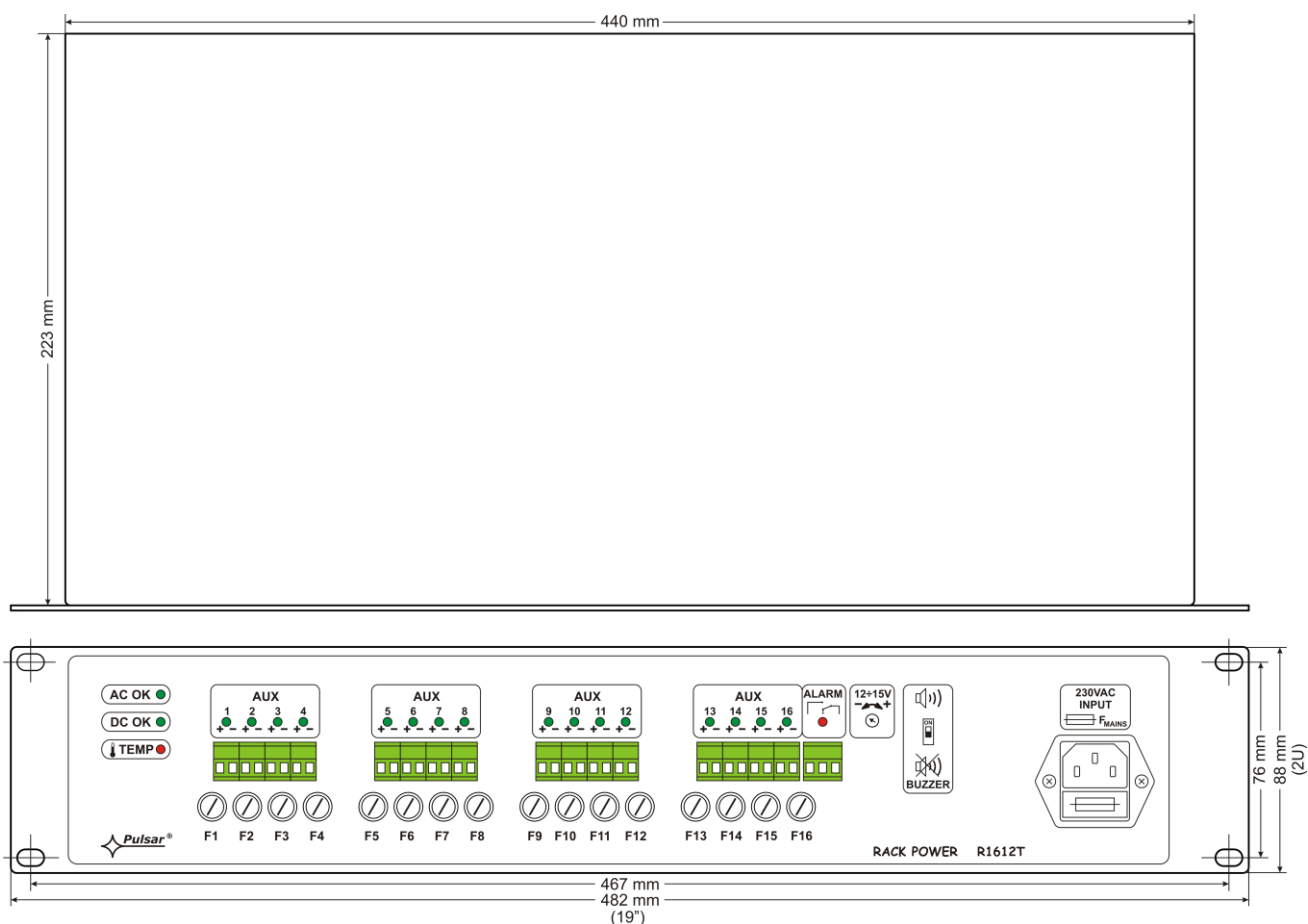
Rys.3. Widok zasilacza.
