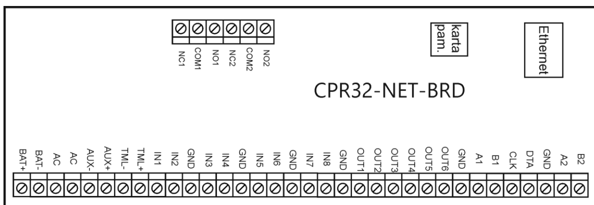
Rys. 1 Centrala CPR32-NET-BRD
