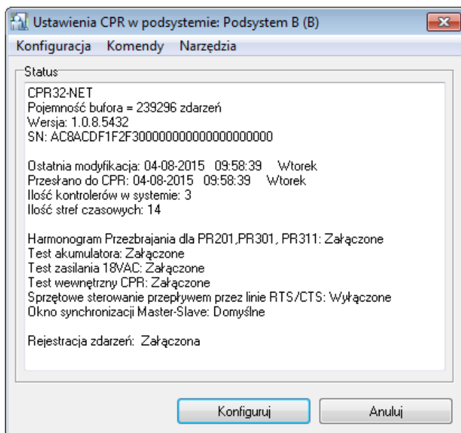
Rys. 9 Opcje centrali CPR32-NET-BRD w programie PR Master
