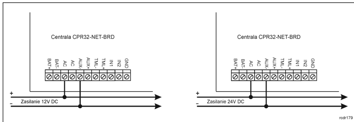
Rys. 4 Zasilanie centrali CPR32-NET-BRD
